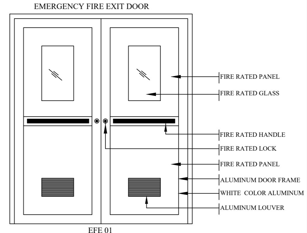
EFE 01 ALUMINUM FRAMED PANELED DOOR
